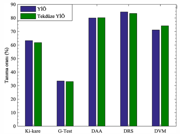
Şekil 6. Sınıflandırma yöntemlerinin YİÖ ve Tekdüze YİÖ için sınıflandırma başarımları.
